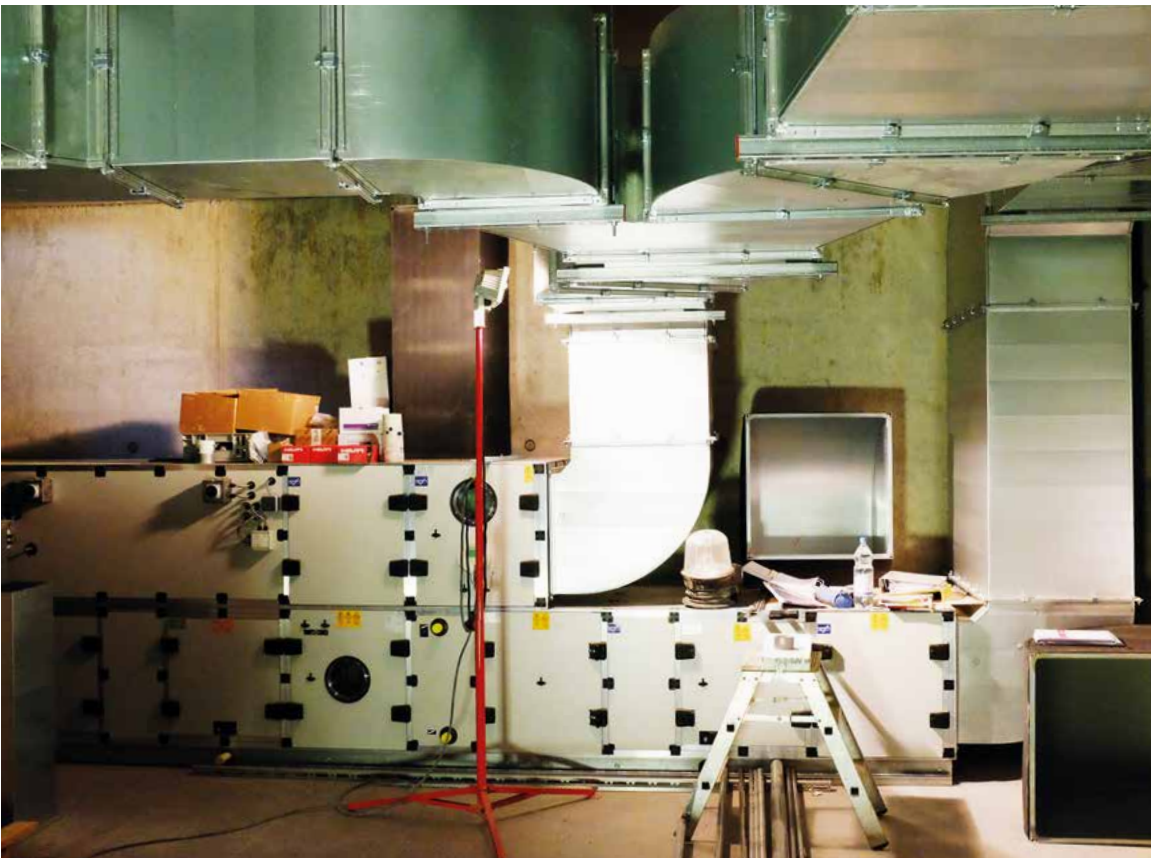
Lüftungsanlage
