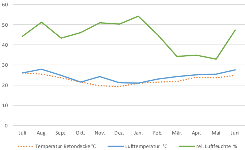
Raumlufttemperatur und Raumluftfeuchte im erweiterten Komfortbereich
