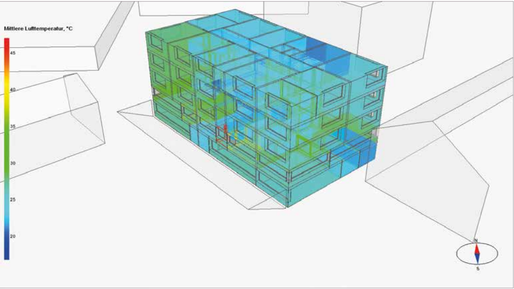
Sommerliche Überwärmung des Gebäudes, dargestellt im Simulationsmodell
