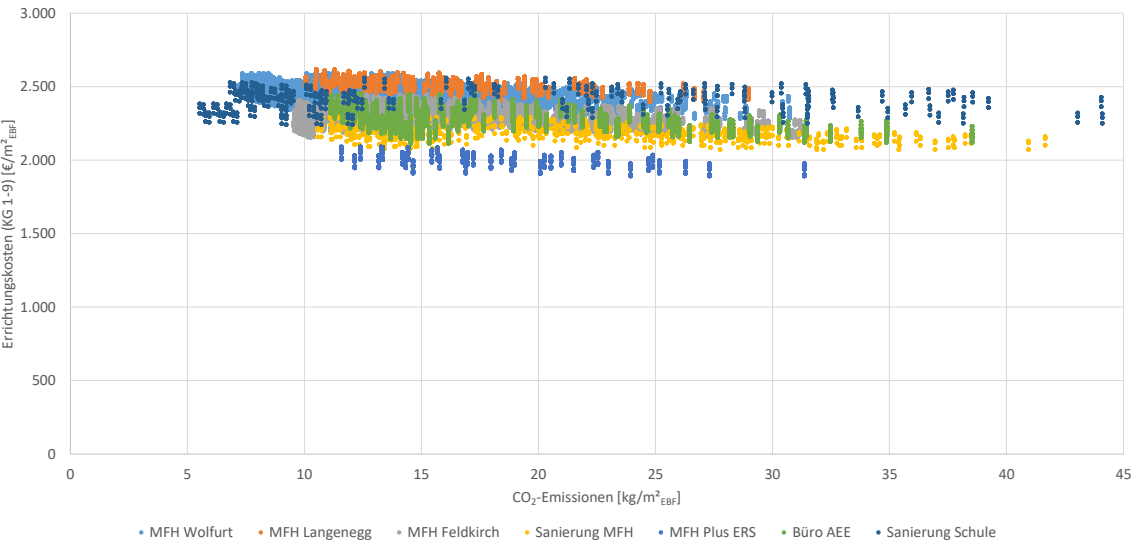
Errichtungskosten (KG 1-9) über den CO 2 -Emissionen der Varianten für alle sieben Beispielgebäude (Bezogen auf Energiebezugsfläche PHPP/ Berechnungen PHPP/ CO 2 -Faktoren OIB RL-6 2015/ keine CO 2 -Gutschrift für eingespeisten Strom)
