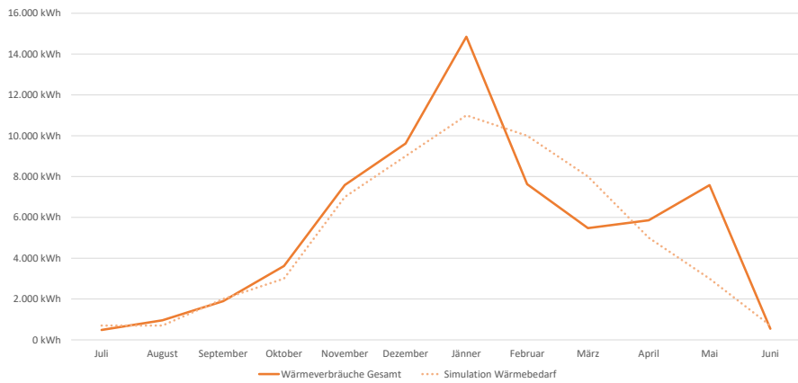
Vergleich Simulation zu Verbrauch
