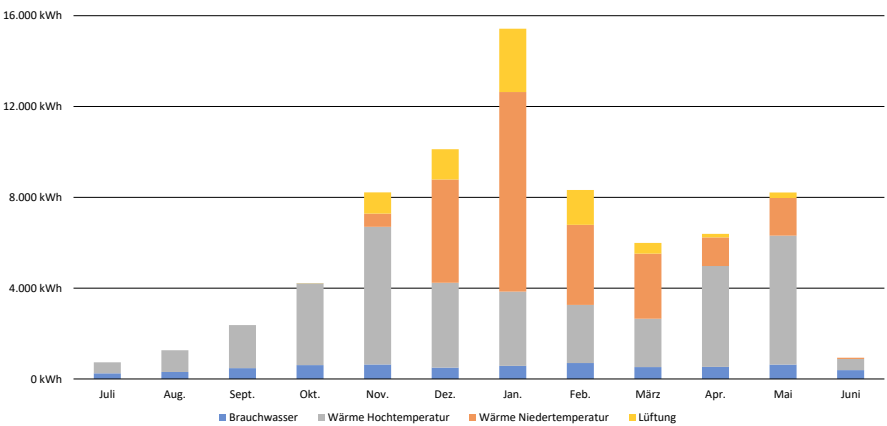
Energieflüsse Wärme
