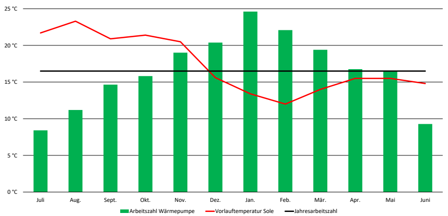
Arbeitszahl Wärmepumpe
