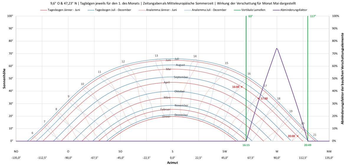
Wirkung von vertikalen Verschattungslamellen, im Sonnenstandsdiagramm dargestellt (grüne Linien)
