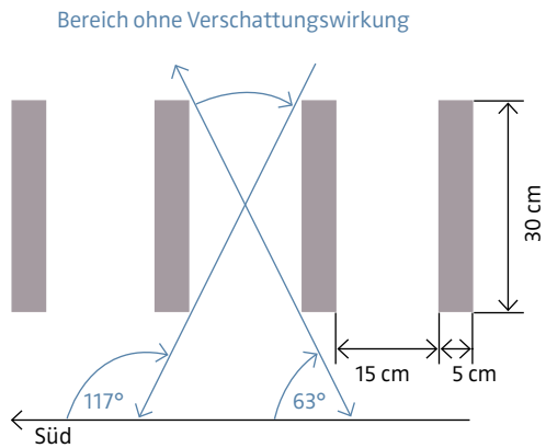
Schema vertikale Verschattungslamellen
