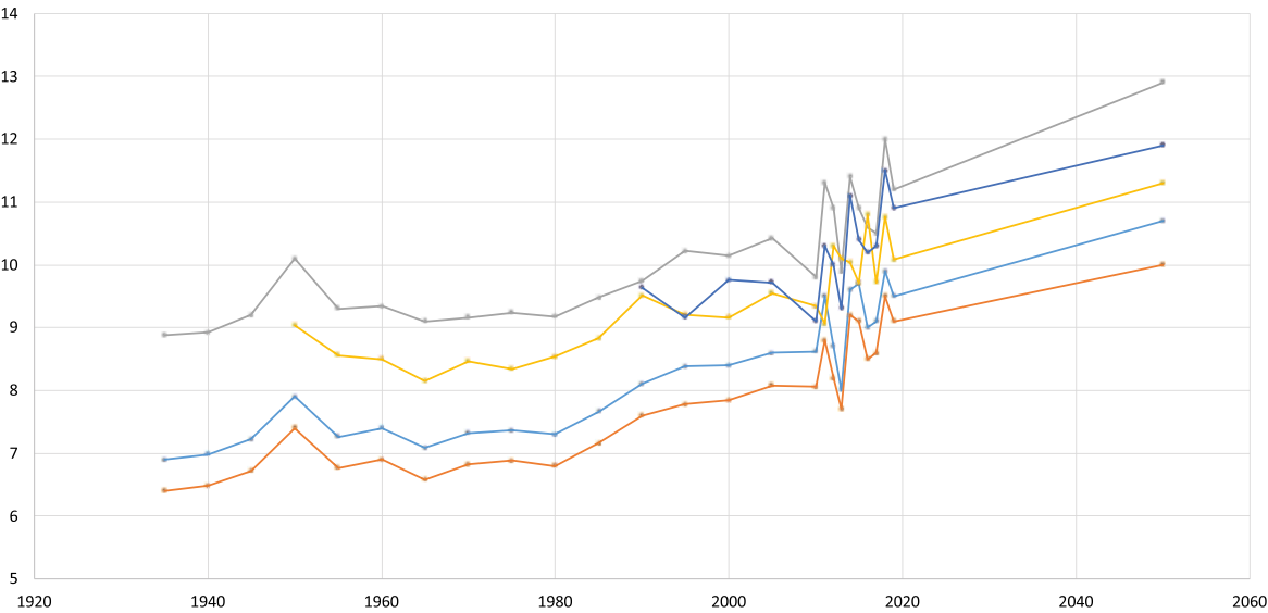
Entwicklung der Jahresmittletemperaturen von 1930 – 2020
