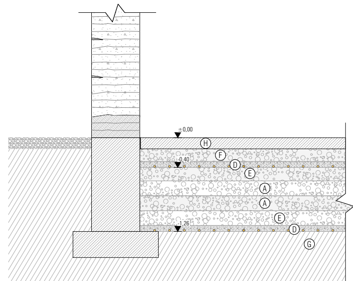
Detailschnitt der zwei Systemaufbauten des Hallenbodens (Anschluss an Stampflehmwand mit Sockel Stampfbeton und Anschluss Maschinengrube/Stampflehmwand)
