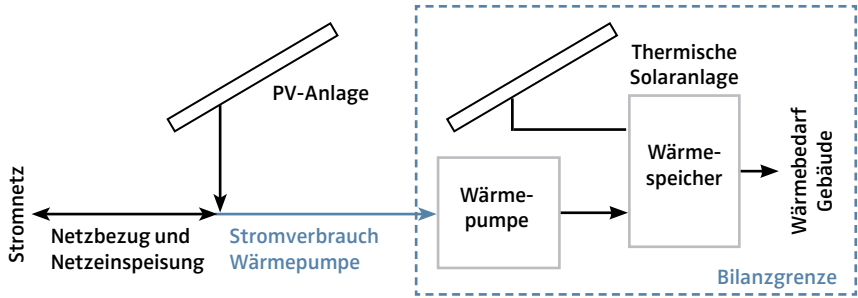
Messbilanz Wärmepumpe
