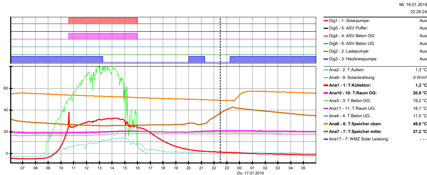
Die Grafik zeigt den Temperaturverlauf über 1,5 Tage im Januar. Die Erträge der thermischen Solaranlage (rote Linie) werden in die thermisch aktivierten Decken eingespeichert. Am Abend wird der Lehm-Grundofen in Betrieb genommen und der Pufferspeicher damit erwärmt (braune und obere rote Linie).
